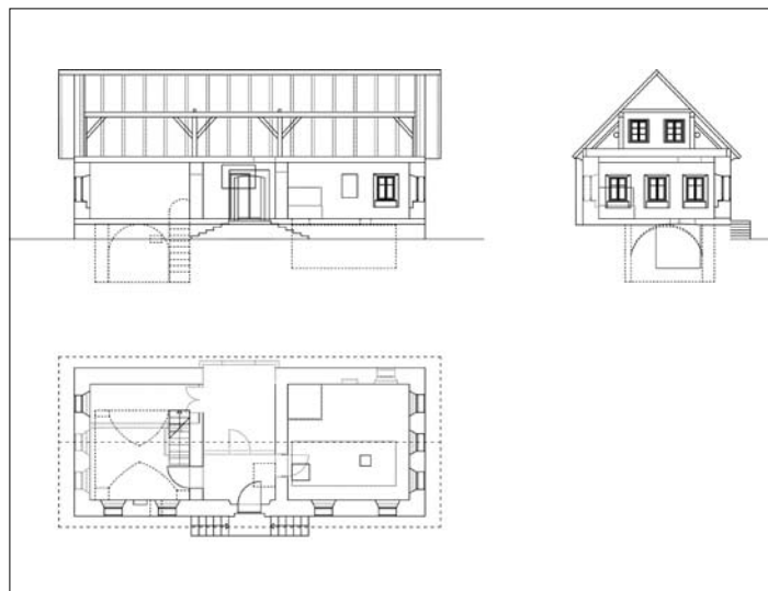
Tloris pritličja Lkčeve hiše, Cesta 49, Nevenka Grm Gregorič, dipl. inž. arh.
